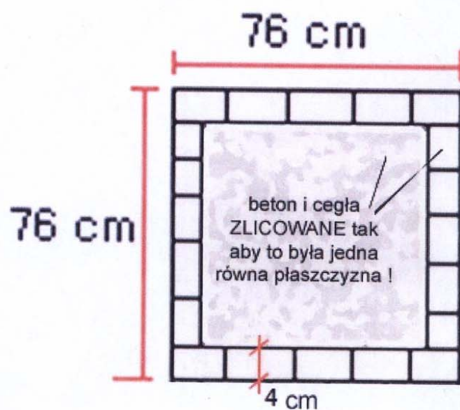
Widok-rzut z góry - podest
